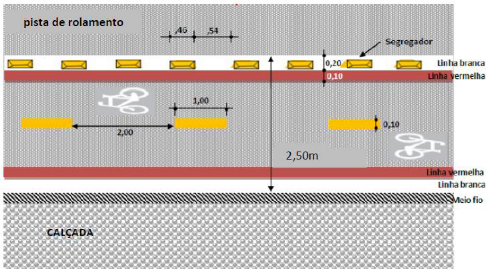
Figura 120 - Ciclofaixa em pista de rolamento compartilhada conforme Caderno de Encargos da PCRJ
