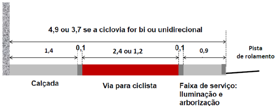
Figura 2911 - Ciclofaixa em calçada compartilhada conforme Caderno de Encargos da PCRJ
