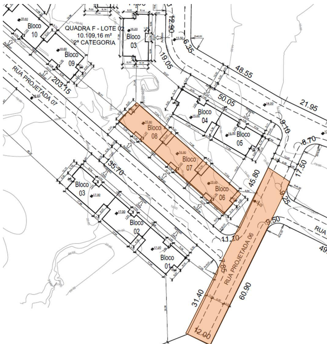
Figura 3 – Identificação dos blocos 06, 07 e 08 do lote 2 da quadra F e da rua projetada 06 do PAA 12767 / PAL 49882 com interferência com benfeitorias existentes
